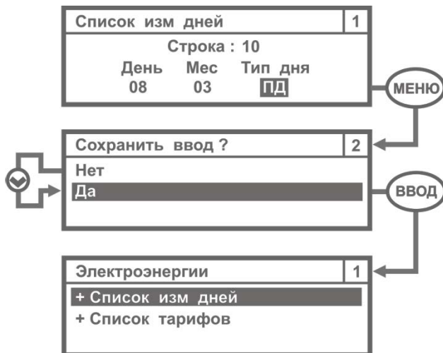
Рисунок 3.31 – Настройка меню Список изменённых дней
