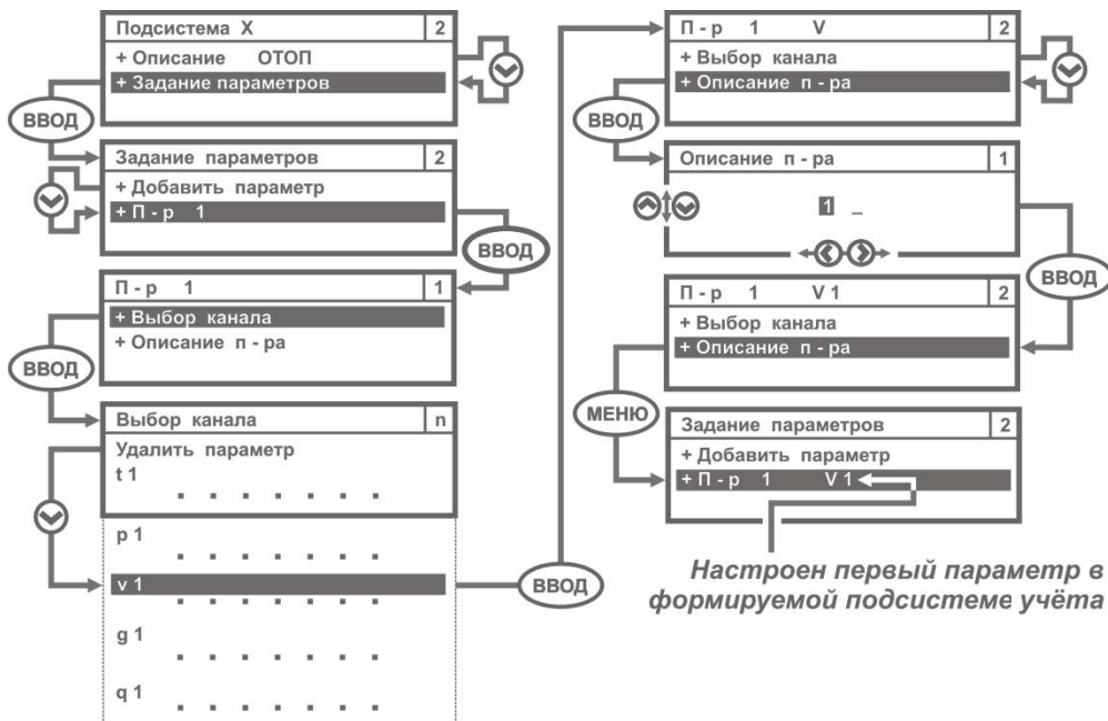
Рисунок 3.38 – Порядок настройки параметров в подсистеме учёта
