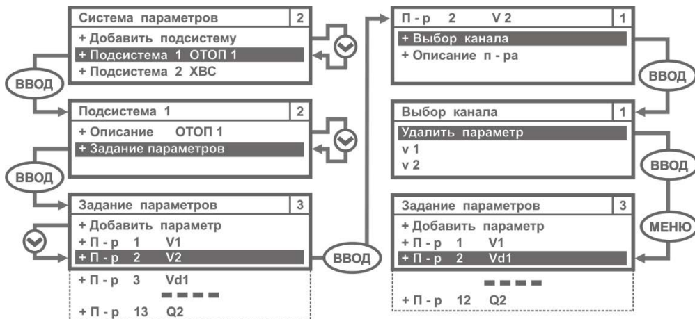
Рисунок 3.41 – Порядок удаления параметров из подсистемы учёта
