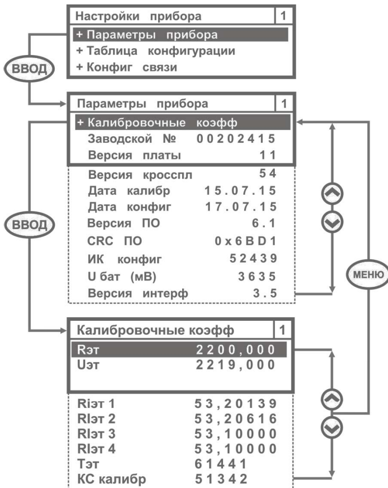
Рисунок 2.1 – Пример развёрнутого изображения меню Параметры прибора
