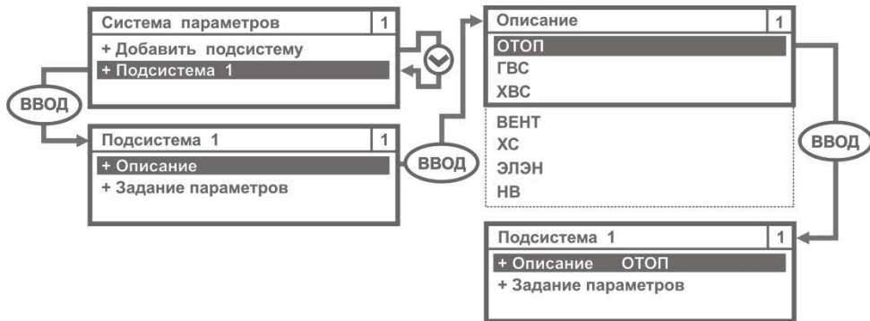
Рисунок 3.36 – Выбор типа первой подсистемы учёта
