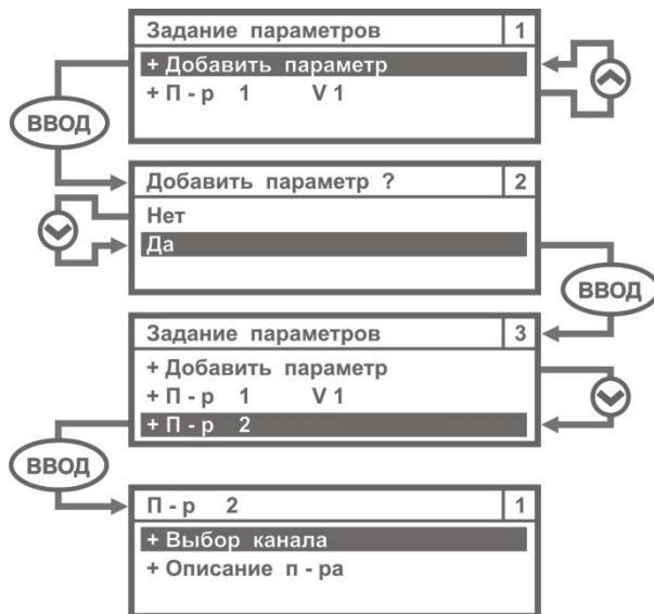
Рисунок 3.39 – Формирование нового параметра для подсистемы учёта
